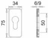
D 812/6MM/F1 SCHUIFROZET 6MM/F1
