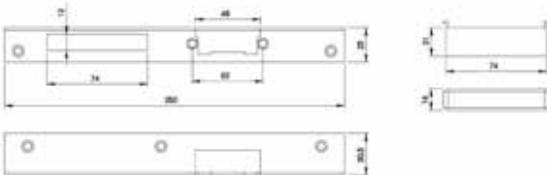
I 033193 VRPL.EL.DEUROP.IN PL KEE NACHT
