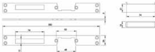
I 033196 VRPL.EL.DEUROP.IN PL.KEER DAGS
