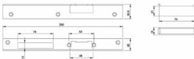
I 033192 HOEKPLAAT GELAKT EL.OPENER DR
