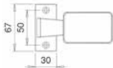
D 315/F1 TREKKER OP ROZET F1
